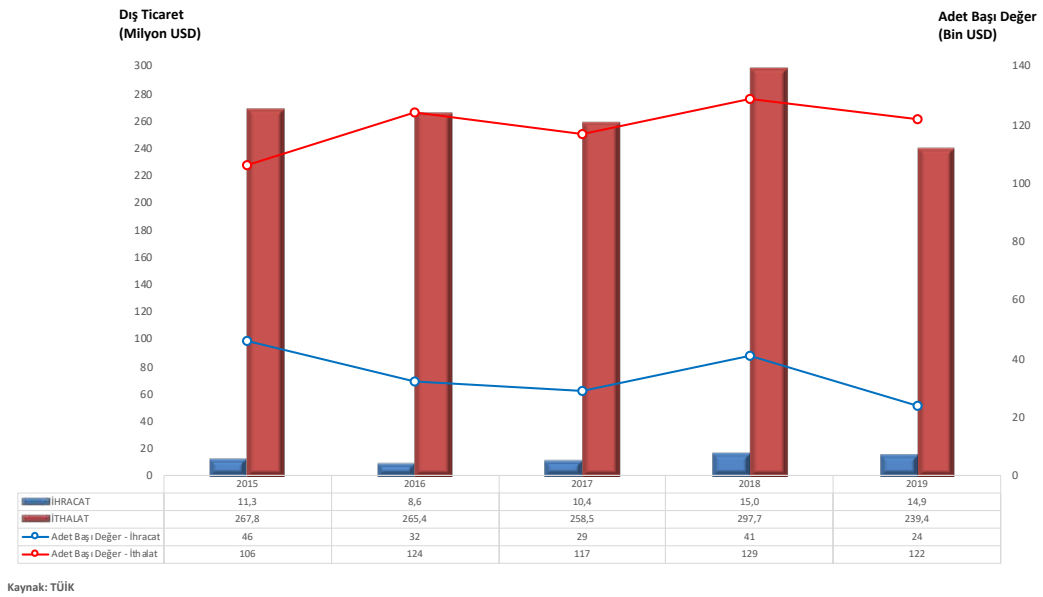
GRAFİK 26: Metal İşlemeye Mahsus İşleme Merkezleri ve Transfer Tezgahları (GTİP 8457)
