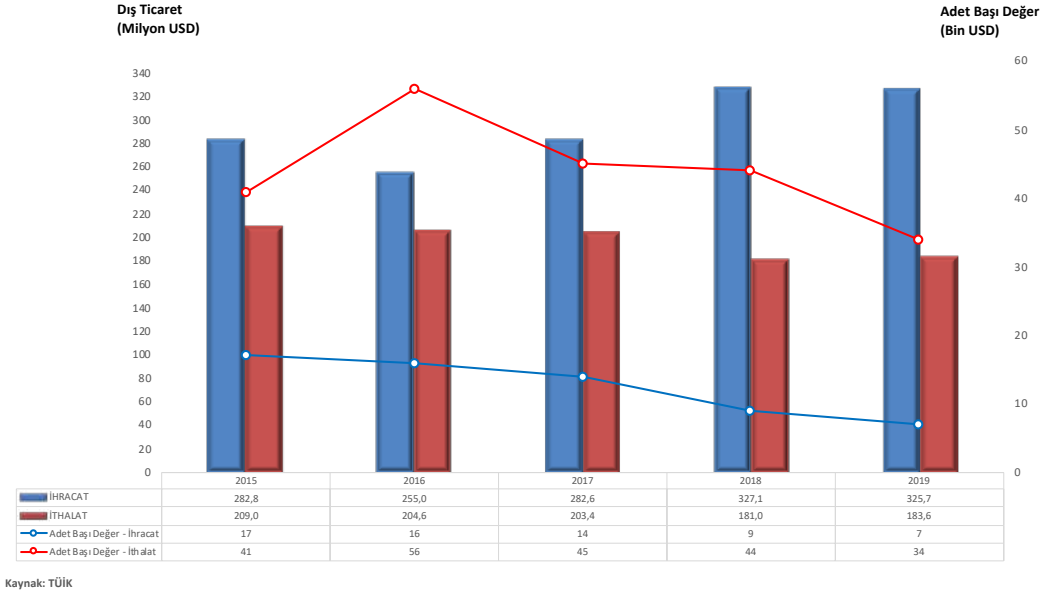
GRAFİK 31: Sac Şekillendirme Tezgahları (Abkant, Panç, Giyotin, vb.) ve Presler (GTİP 8462)
