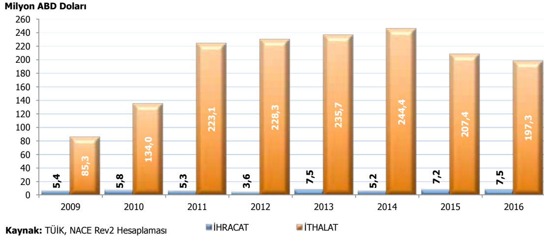
GRAFİK 29: Metal İşlemeye Mahsus Torna Tezgahları (Tornalama Merkezleri Dahil) (GTİP 84.58)
