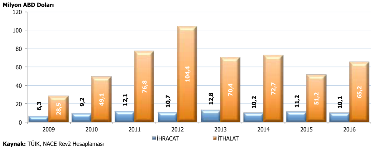
GRAFİK 30: Metalleri Talaş Kaldırmak Suretiyle Delmeye, Raybalamaya, Frezelemeye, Diş Açmaya Vb Mahsus Takım Tezgahları (GTİP 84.59)
