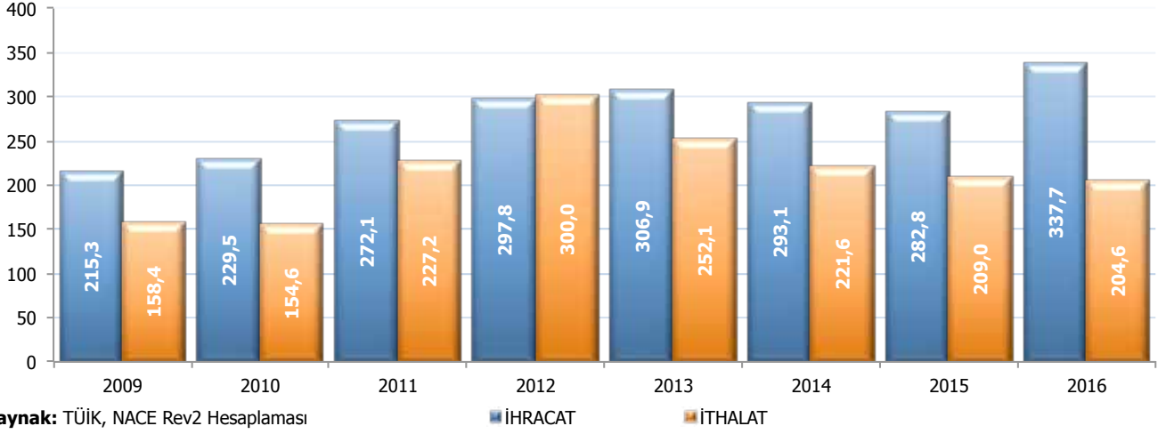
GRAFİK 33: Metalleri Dövme, Çekiçleme, Kalıpta Dövme, Kesme, Taslak Çıkartma, Şatafatlama, Karbürleri İşlemeye Mahsus Takım Tezgahları (GTİP 84.62)
