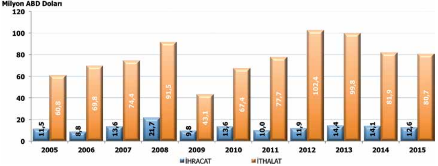
GRAFİK 32: METALLERİ VEYA SERMETLERİ PARLATMA, ÇAPAK ALMA, BİLEME, TAŞLAMA, HONLAMA, LEPELEME, PARLATMAYA VB MAHSUS TEZGAHLAR (GTİP 84.60)
