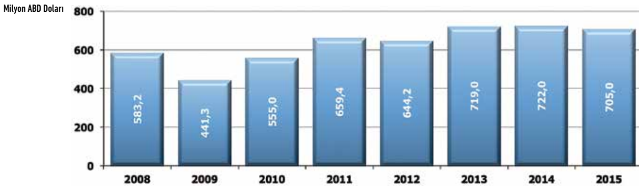
GRAFİK 7: YILLARA GÖRE TAKIM TEZGAHLARI İMALATI, TÜRKİYE
