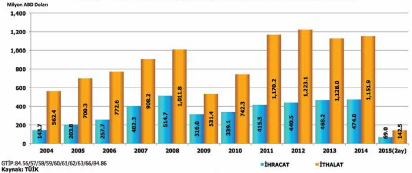
Grafik23: TAKIM TEZGAHLARI; Metal İşleme Makineleri Dış Ticareti (NACE 2: 28.41)
